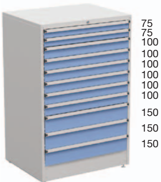
Höhe 1400 mm
