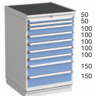
Höhe 1100 mm
