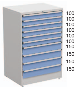
Höhe 1400 mm
