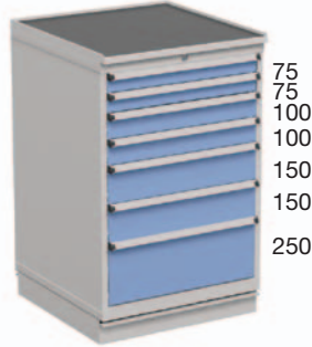
Höhe 1100 mm
