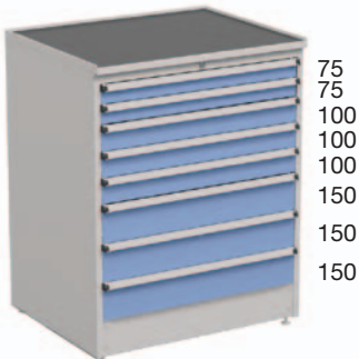
Höhe 1100 mm
