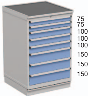
Höhe 1100 mm
