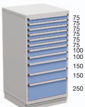
Höhe 1400 mm
