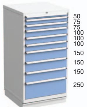
Höhe 1400 mm
