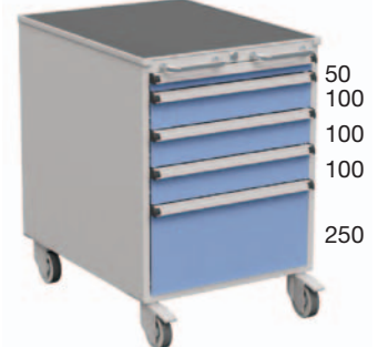
Höhe 795 mm
