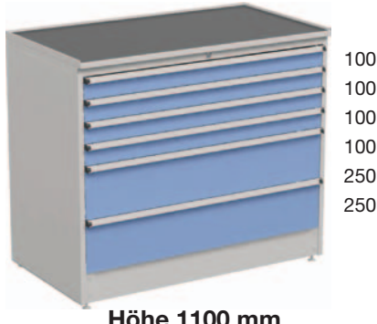
Höhe 1100 mm
