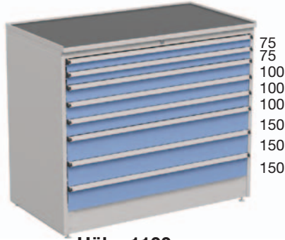
Höhe 1100 mm
