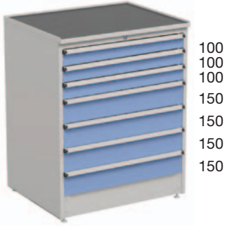
Höhe 1100 mm
