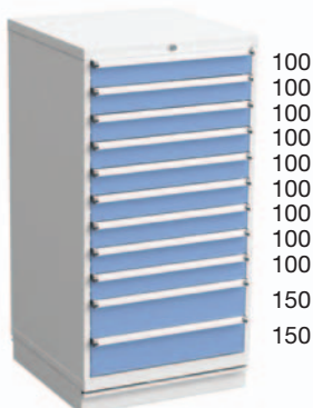
Höhe 1400 mm
