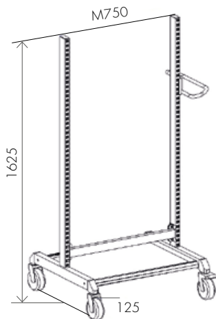
Basic-Wagen, Gestell
